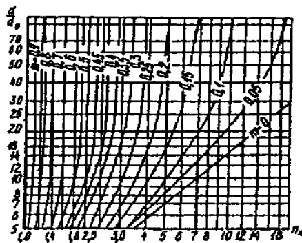
Рисунок 2 – Номограмма для определения начального разбавления в потоке
